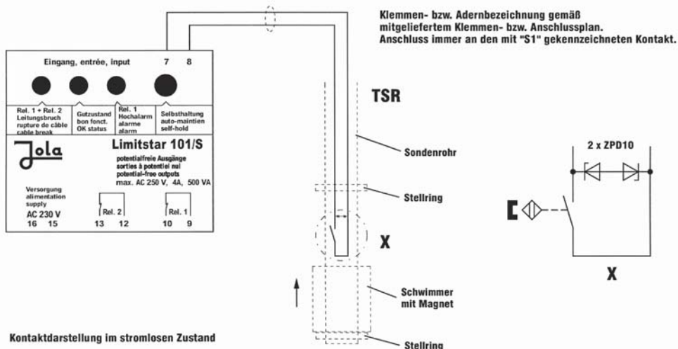
Bild: Elektrischer Anschluss Standaufnehmer/Messumformer
