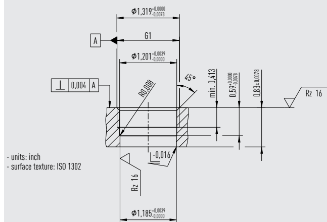
G 1 flash
