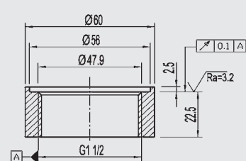
G 1 ½ 1)
