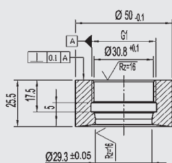
G 1, EHEDG 1) 2) 3)
