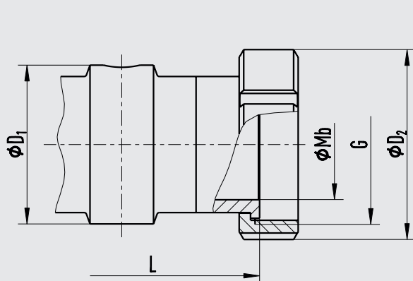
Union nut (SS 1148)
